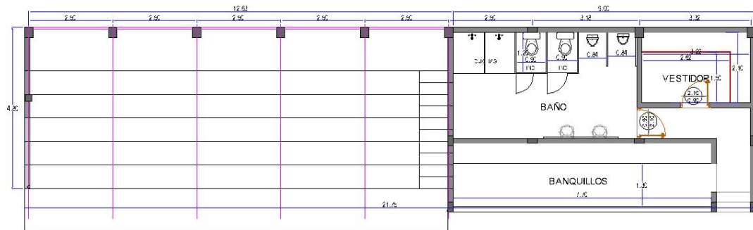
PLANTA GRADA CON DOGAUT Y BAÑOS RIGHT FIELDER
