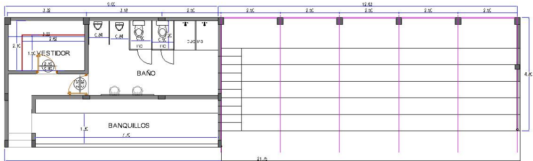
PLANTA GRADA CON DOGAUT Y BAÑOS LEFT FIELDER
