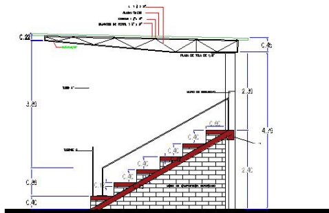
SECCION TRANSVERSAL
